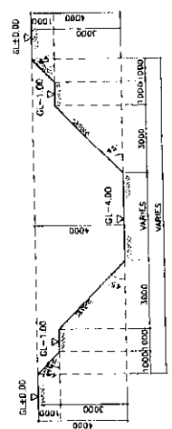
รูปตัด (1) แสดงระดับจุดบ่อน้ำ (1) ขนาดย่อ 1:100
